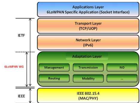
Fig. 5. 6lowpan adaptation layer
